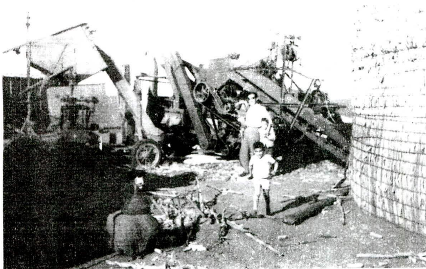
Desgranadora de maíz c/motor propio.
